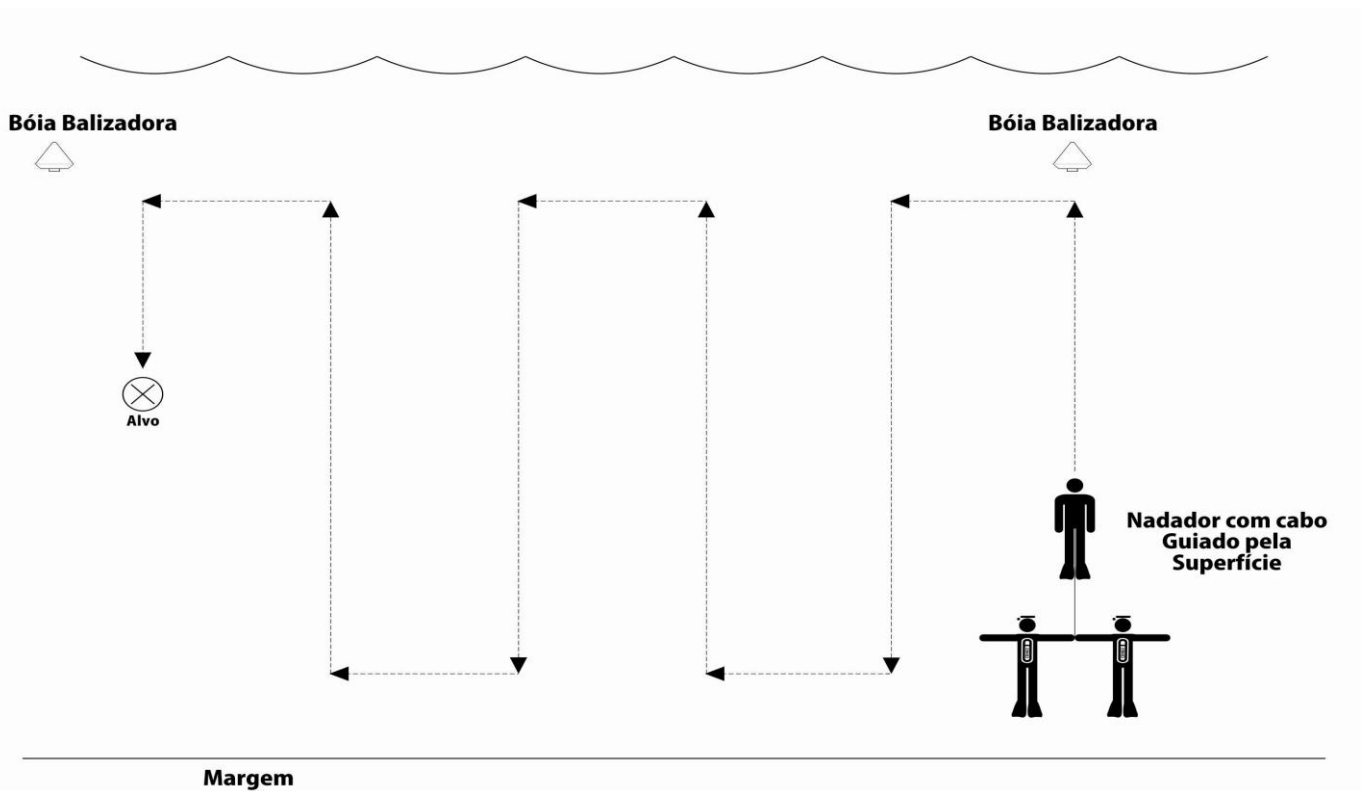
Figura 09 – Varredura em "U", com cabo guiado por nadador na superfície.
