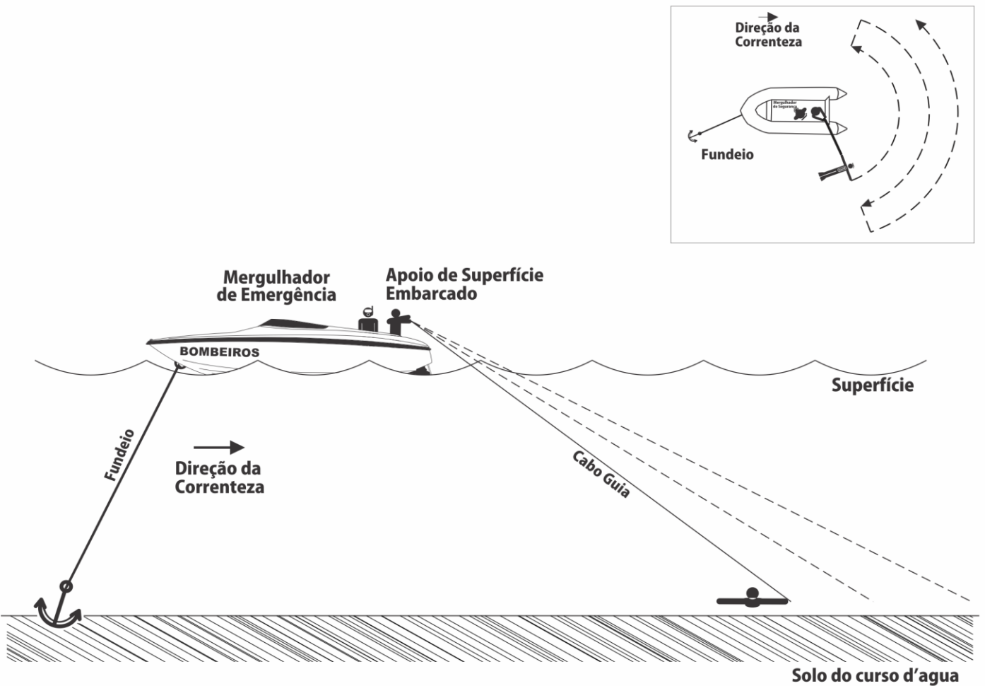
Figura 05 – Busca semicircular com Apoio de superfície embarcado.
