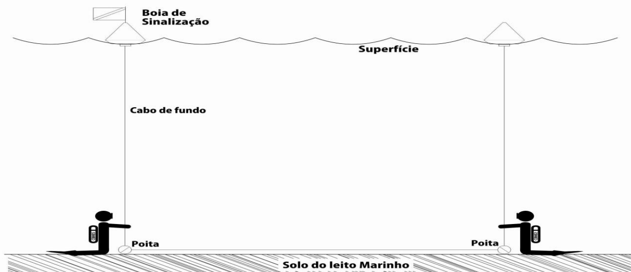
Figura 07 – Esquadrinhamento sem Apoio de superfície na margem.
