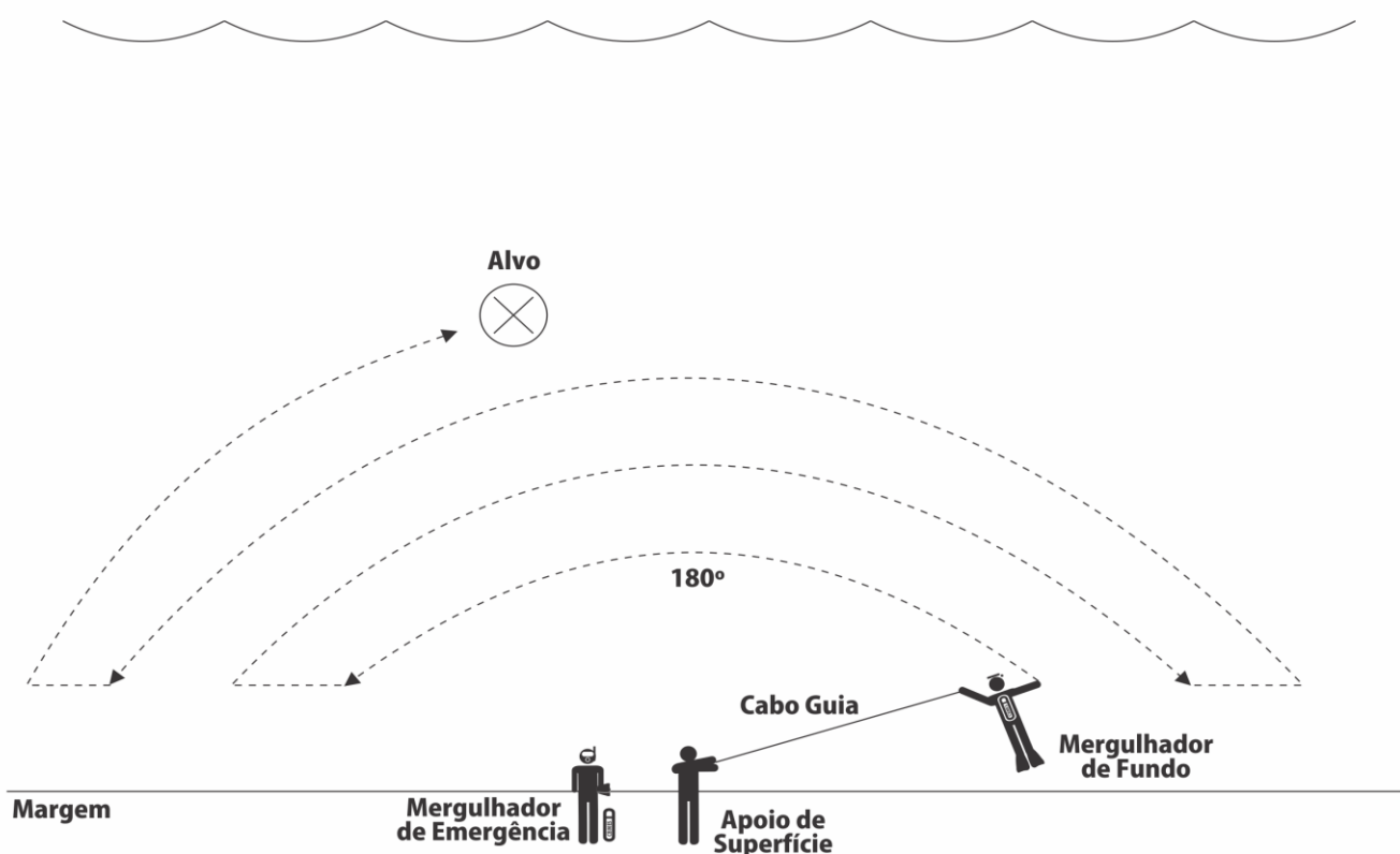
Figura 04 – Busca semicircular com Apoio de superfície a partir da margem.
