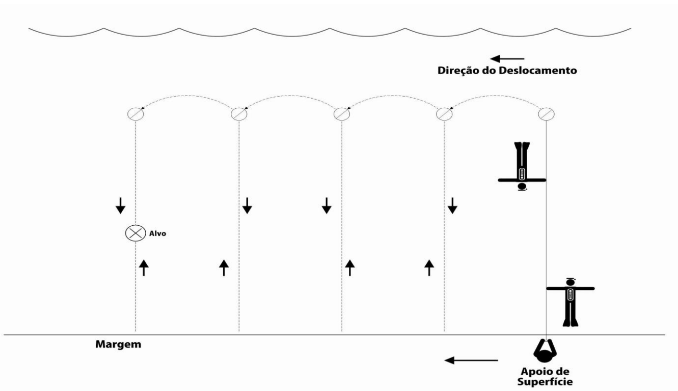
Figura 06 – Esquadrinhamento com Apoio de superfície na margem.
